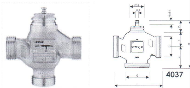
Slika 1. Izgled i dimenzije ventila HERZ kataloški br. 1 4037 xx
